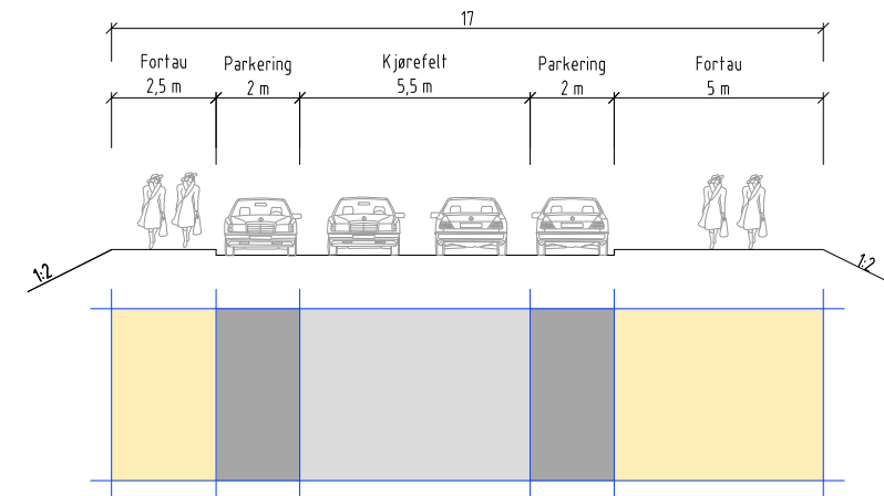
Snitt 18-18 Brekkeveien
