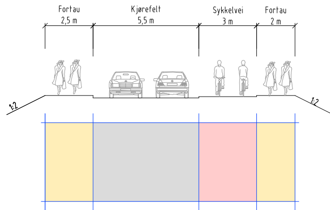
Snitt 15-15 Brekkeveien, Sykkelvei med fortau
