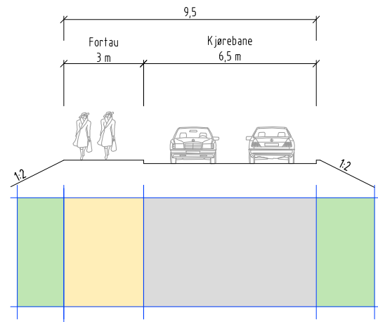
Snitt 10-10 Fv152 Drøbakveien
