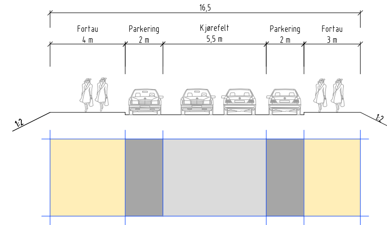
Snitt 17-17 Brekkeveien
