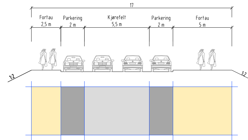
Snitt 18-18 Brekkeveien
